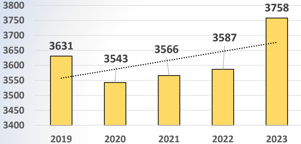
VWU Cases
